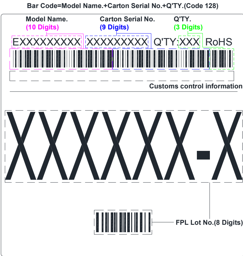
Carton Label
